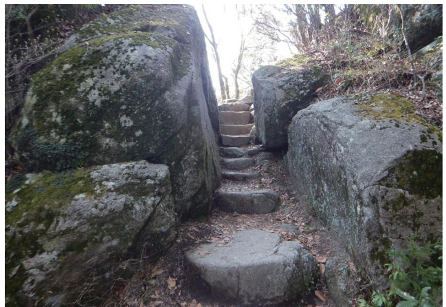
写真 3-10 袖すり岩
