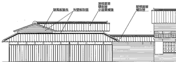
北立面図
