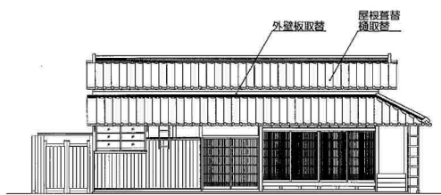
東立面図
