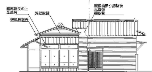
西立面図
