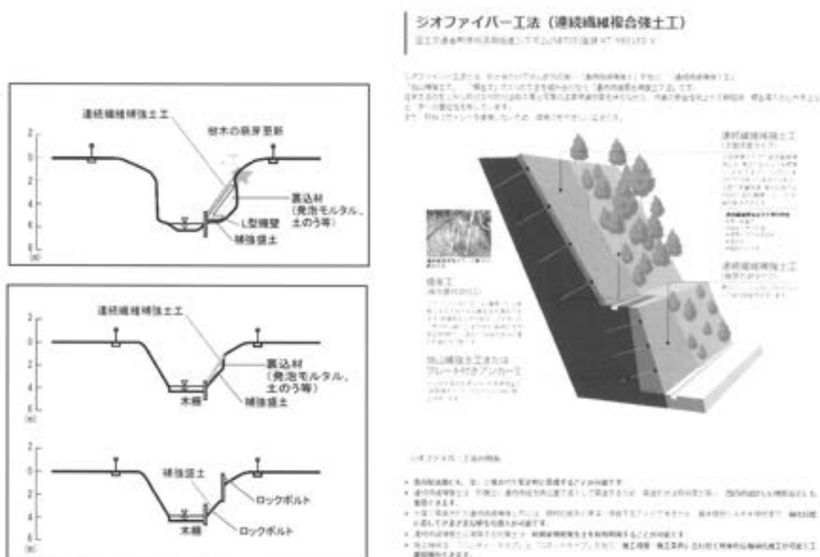
図6-3：表層崩壊の修復イメージ（参考：史跡玉川上水保存管理計画書）
