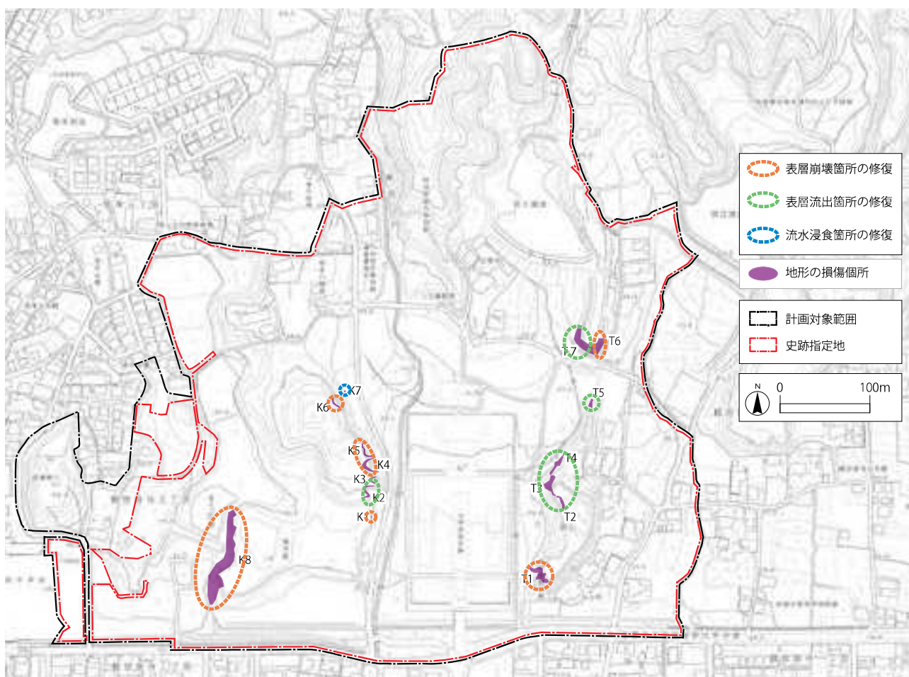
図6-2：地形の造成に関する整備計画
